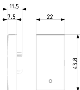
09005.0.250 - 1P 16AX 2- way switch mech.+pilot250V
